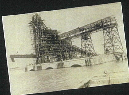
↑ No.7 内港載炭機組立
