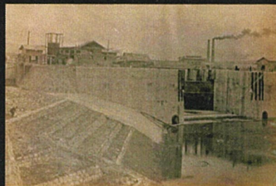
↑ No.4 外側より閘門を望む
