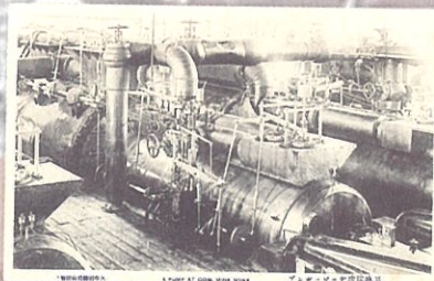
▼三池炭坑デービーポンプ(絵葉書)
